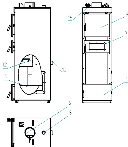
Рис.2 Котлы KC-T -50...
