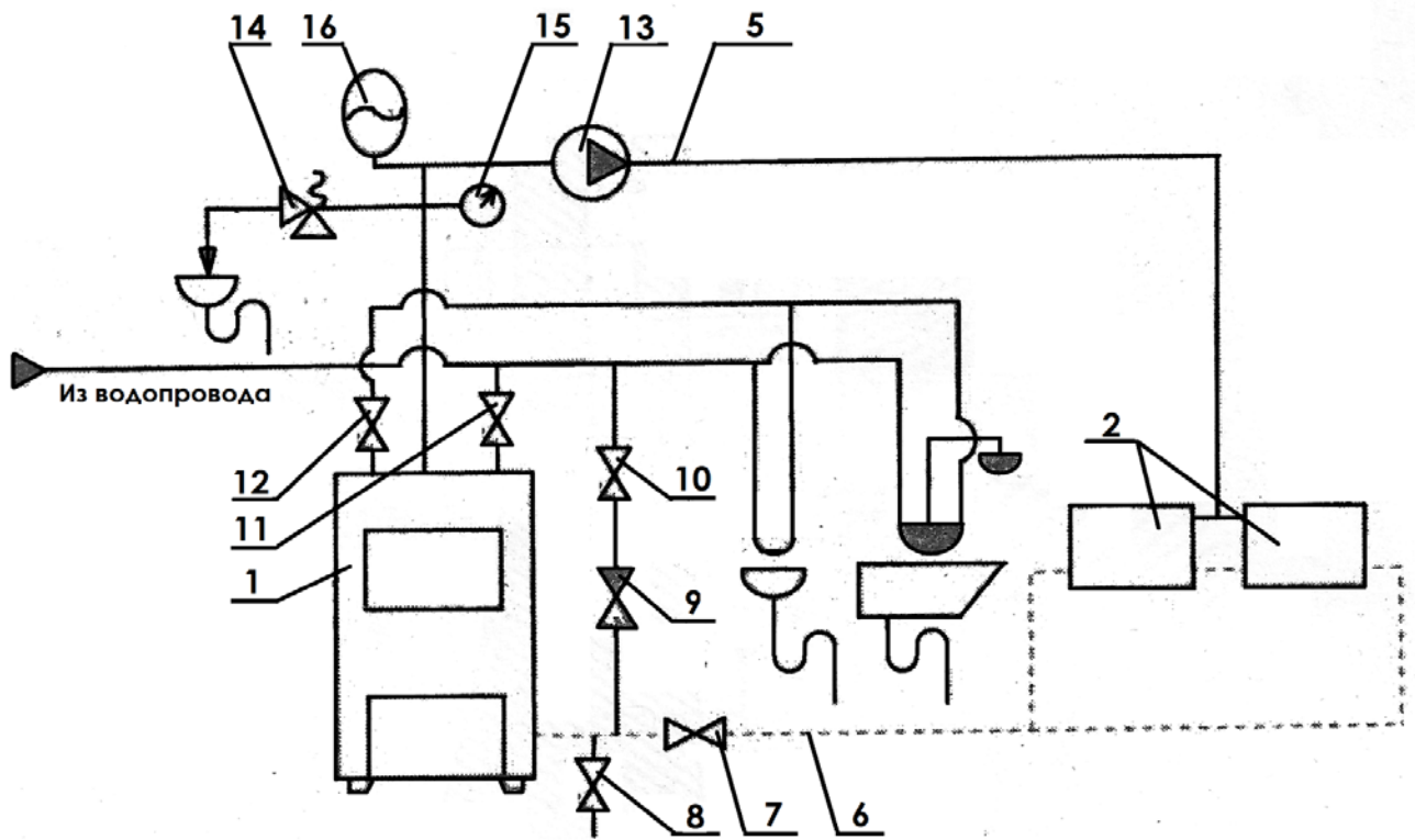
Закрытая система отопления.
