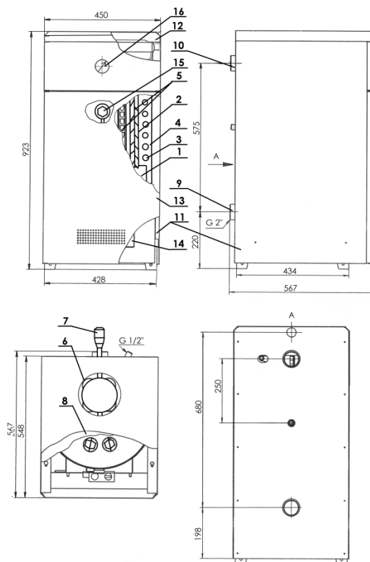
Рис.2 Котел КСЦ-Гм/ГВм-20/25/31,5...
