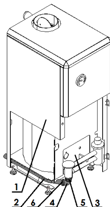
КСЦ-Г/ГВ-10/12/16Н
