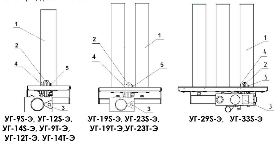
Рис. 4 Газогорелочные устройства с автоматикой безопасности и регулирования.
