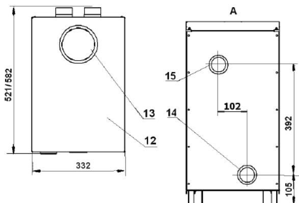
Рис.2 Котлы KC-Г-16S-Э/20S-Э/16T-Э/20T-Э Остальное см. рис. 1
