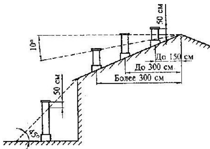
Схема вывода дымовых каналов на крышу здания
