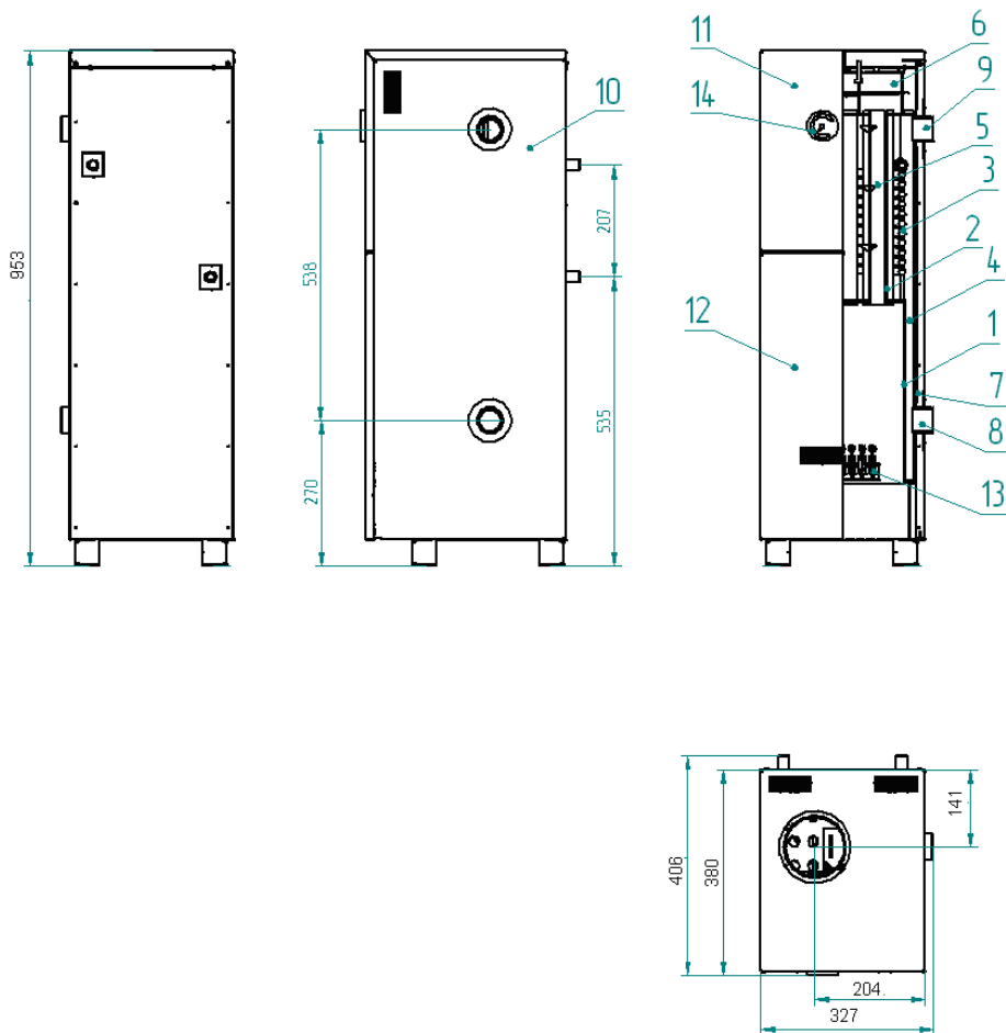
рис.1 Аппараты АОВГ/АОВГК -11,6-1
