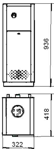
рис.4 Аппараты АОГВ/АОГВК -11,6-3-2 Остальное см. рис.2
