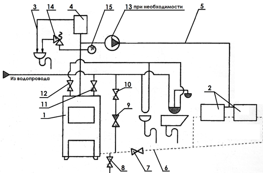
Открытая система отопления
