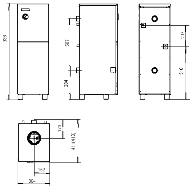
рис.2 Аппараты АОГВ/АКГВ -11,6-3. Остальное см. рис. 1
