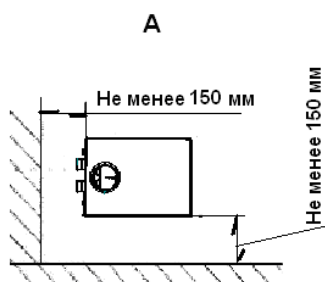
Схема установки аппаратов
