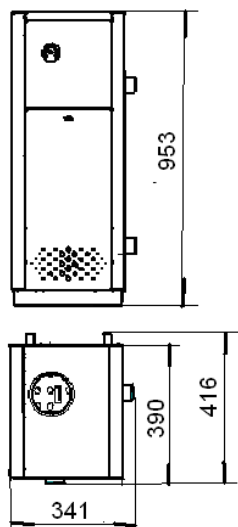
рис.3 Аппараты АОГВ/АОГВК -11,6-1-2 Остальное см. рис. 1
