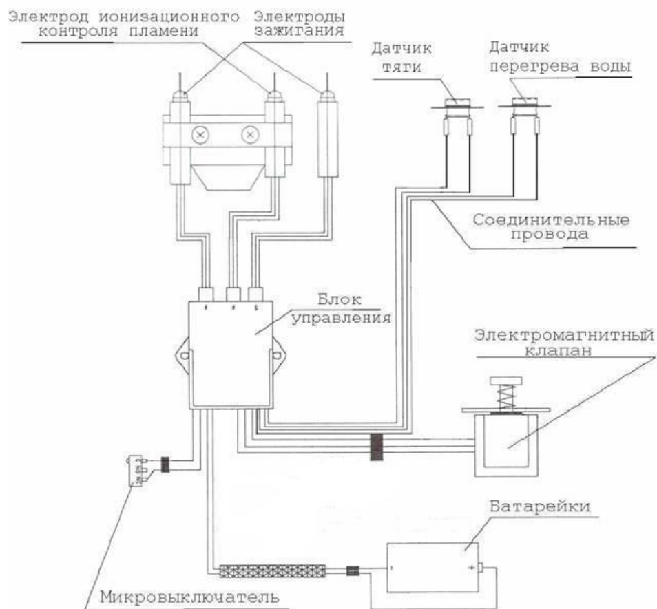
Рис. 2. Схема электрическая
