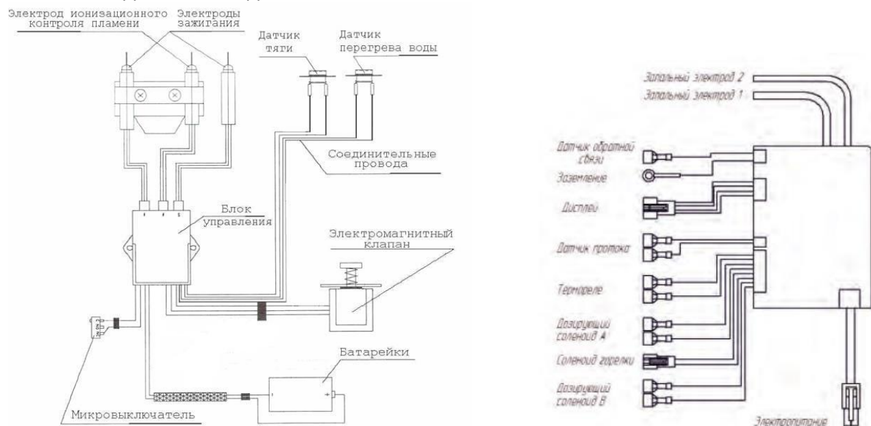
Рис. 2. Схема электрическая
