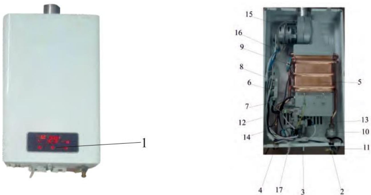
Рис. 2.1 Модель Дон-JSD20-FT
